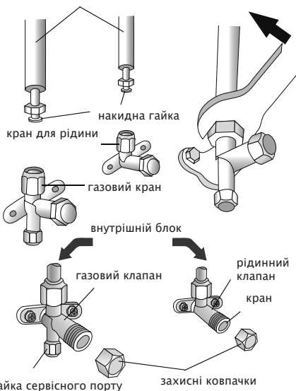
з'єднувальні труби
