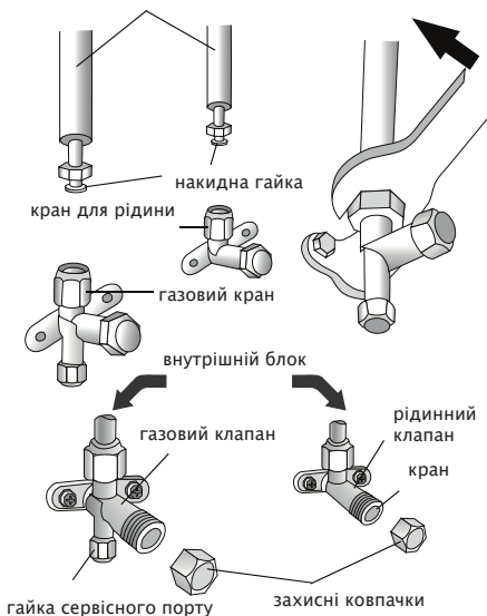
з'єднувальні труби
